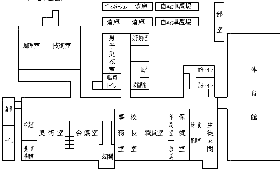
(一階平面図)
