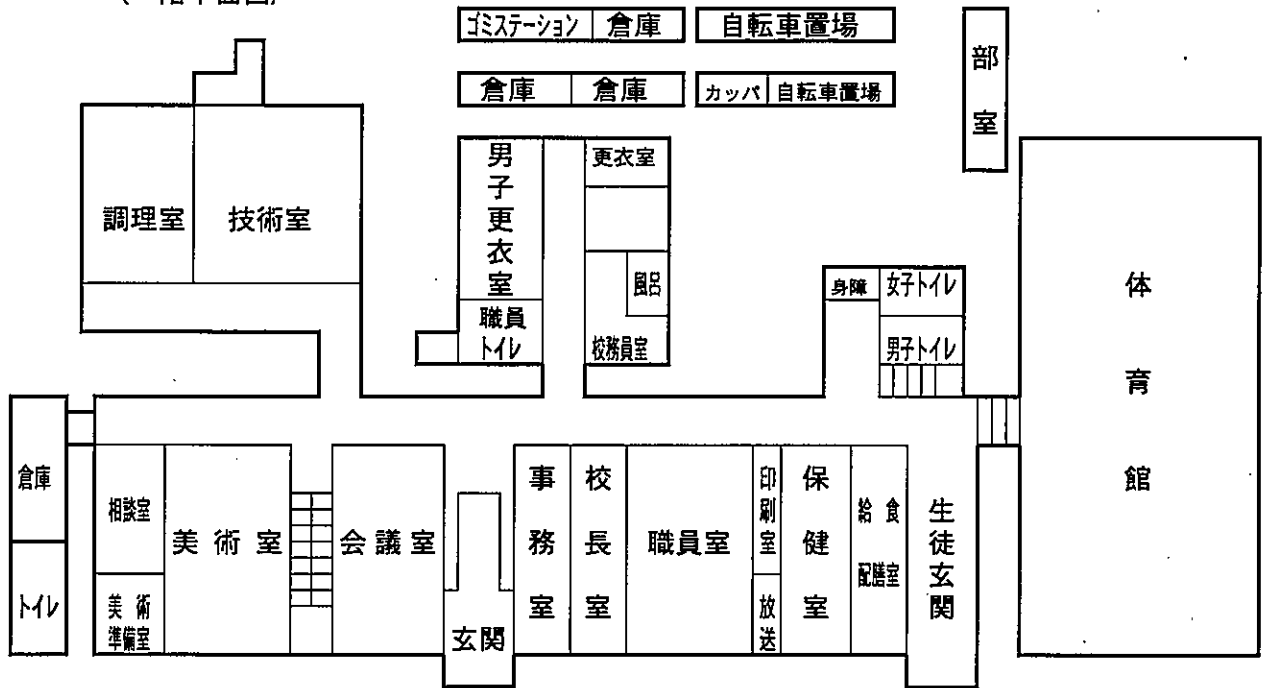
(一階平面図)
